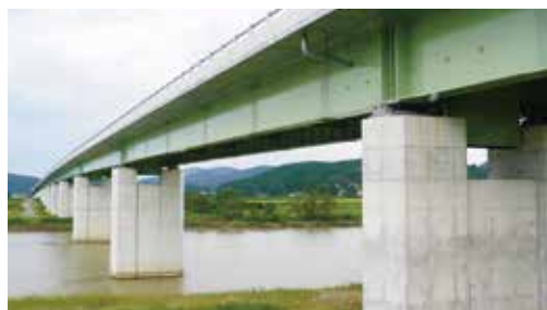
鋼連続2主桁橋
